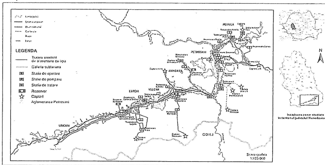
Figura 3-1 Zona de alimentare cu apă în Valea Jiului
